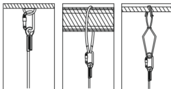
Unión de la cuerda de trabajo a un punto de la estructura fija
