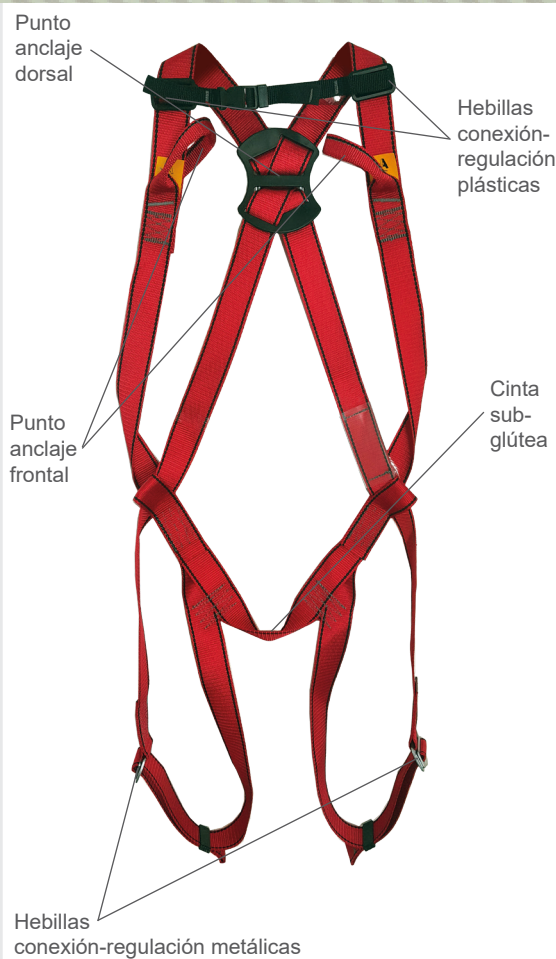
Vista frontal del arnés de seguridad A03S
