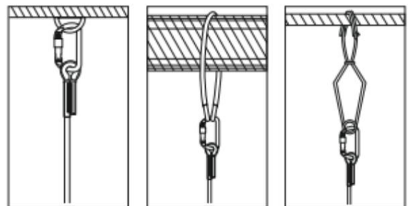
Fissaggio della fune di lavoro ad un punto fisso della struttura
