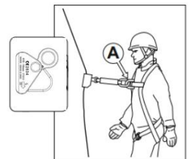
Fissaggio del dispositivo a un'imbracatura di sicurezza
