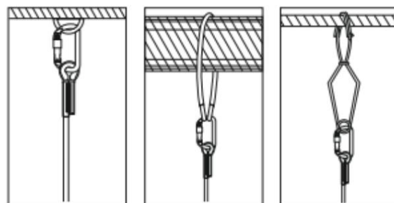
Fixação da corda de trabalho a um ponto fixo na estrutura
