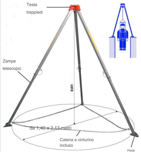
Treppiede TRI 9
